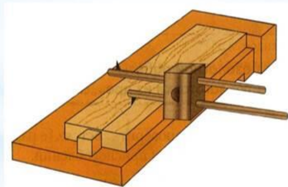
Разметка при помощи рейсмуса
